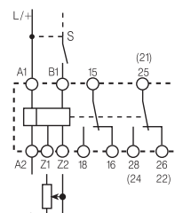
Схема электрических соединений (с сигналом START)
