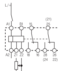
Схема электрических соединений (без сигнала START)
