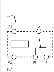
Схема электрических соединений (без сигнала START)
