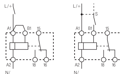
Схема электрических соединений (без сигнала START)
