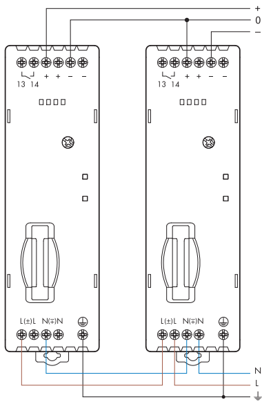
Соединение с двойной полярностью
