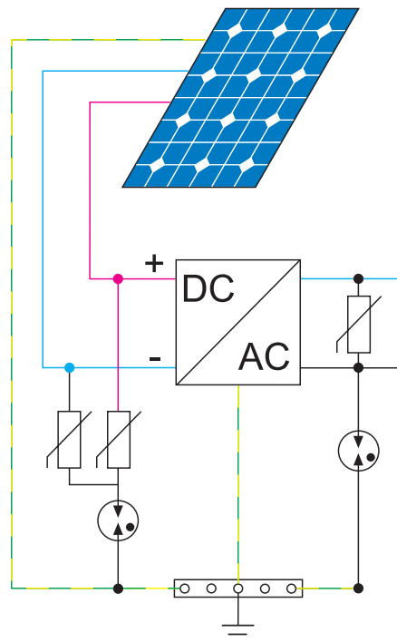
Рис 10: Пример фотогальванической системы для здания, не оборудованного системой защиты от молний; защита со стороны DC при помощи УЗИП с U_{OCSCT} = 420 В, и защита со стороны AC устройством 7P.22, характерным для систем TT.
