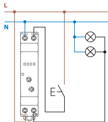
Тип 15.21 - 4-проводное соединение
