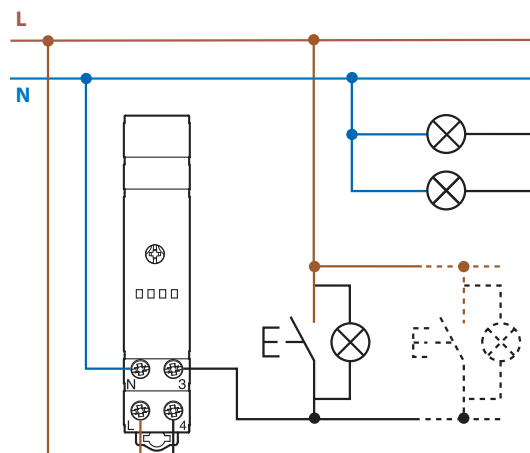
4-проводное соединение
